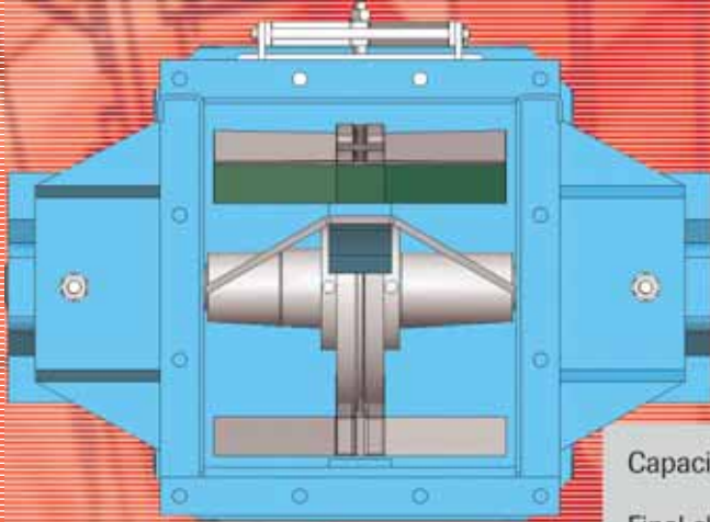
A-A (1:5)
